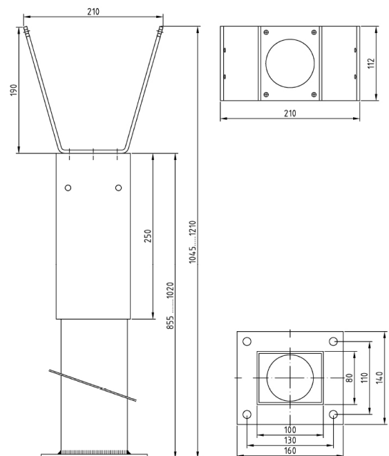
Verstelbare vangpaal met magneet
