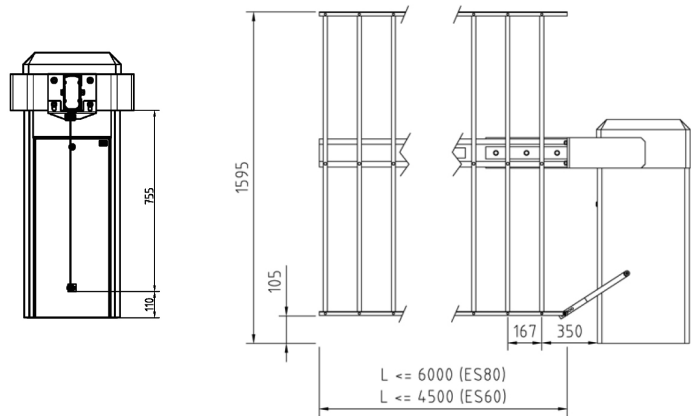
Schaarhek 150
