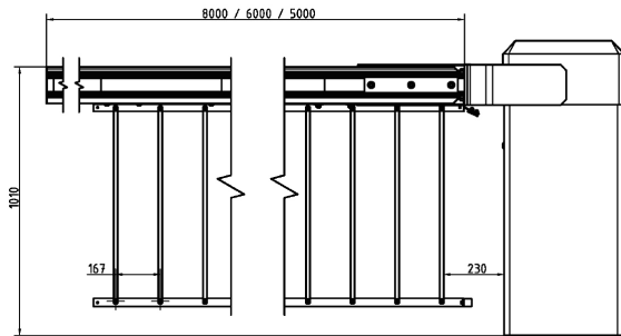
Schaarhek 75
